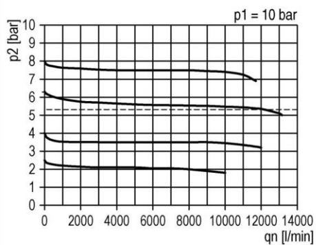
Durchflussdiagramm
